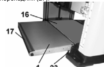
Рис. 5 (вид спереди)
