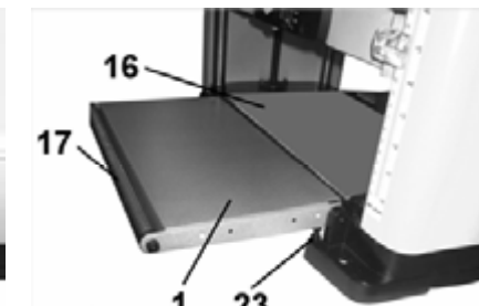
Рис. 6 (вид сзади)
