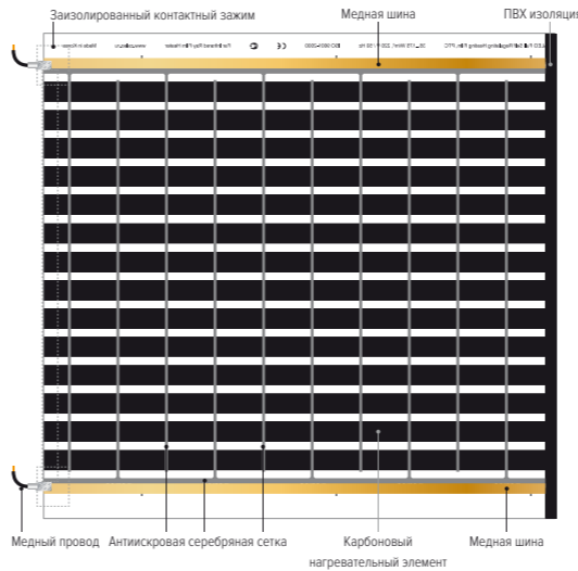
Рис. Общий вид термоленты CALEO, расположение основных ее элементов, контактных зажимов и мест подключения и изоляции
