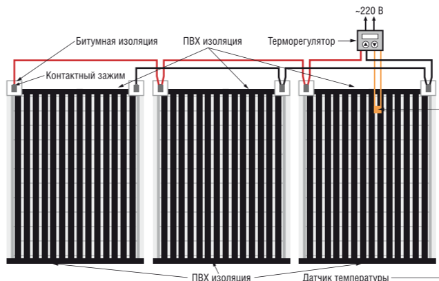
Закрепленный контактный зажим
