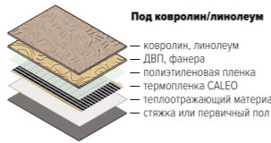
Рис. Схема монтажа теплого пола CALEO под ковролин или линолеум
