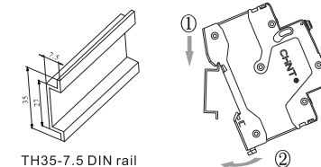
TH35-7.5 DIN rail
