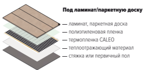
Рис. Схема монтажа теплого пола CALEO под ламинат или паркетную доску
