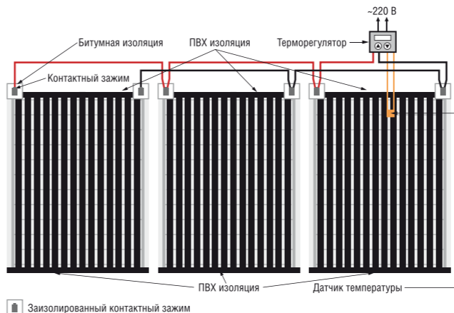
Рис. Общая схема подключения термоленты CALEO PLATINUM
