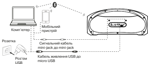
Мал. 4. Схема підключення
