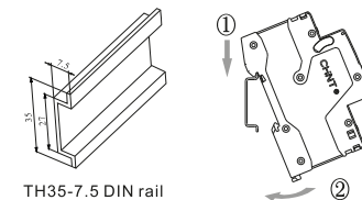
TH35-7.5 DIN rail
