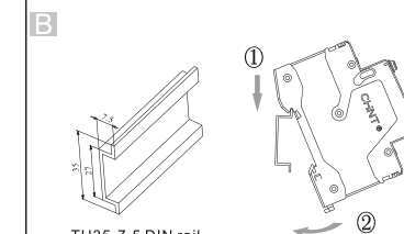
TH35-7.5 DIN rail
