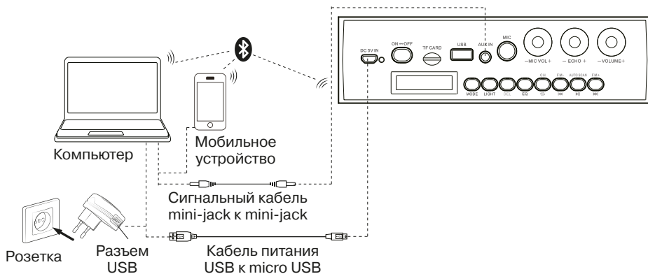
Рис. 2. Схема подключения
