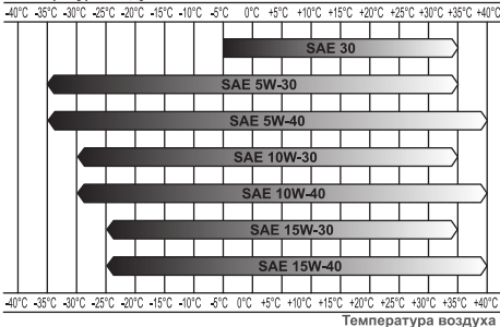
Рис.15 Таблица выбора моторного масла
