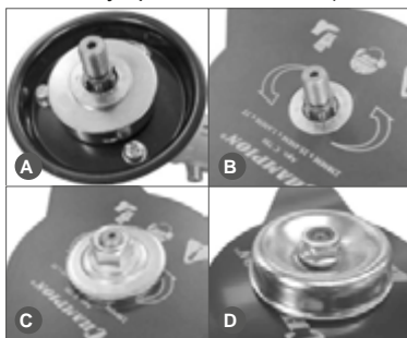
Рис. 5 Установка ножа
