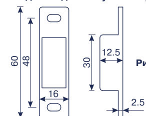
Вкладыш под ответную планку
