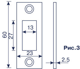
Ответная планка
