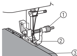
1 Винт 2 Направляющая 3 Подогнутый край
