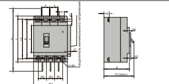
Габаритные и установочные размеры автоматических выключателей NM1-63, 125, 250
