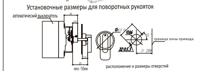
Установочные размеры для поворотных рукояток
