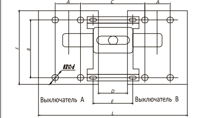
Установочные размеры механической блокировки
