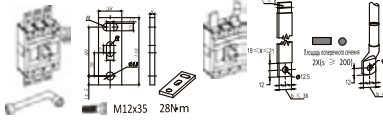
NM1-630 размеры шинных выводов и подключаемого проводника
