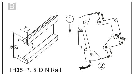
TH35-7.5 DIN Rail
