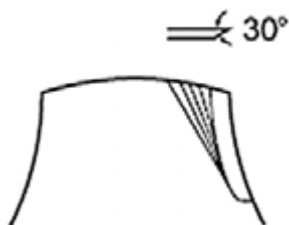
Рис. 19 Заточка ножа
