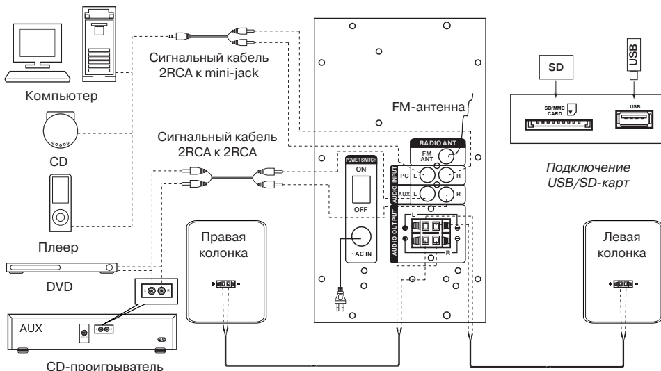
Рис. 4. Схема подключения
