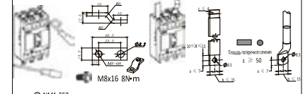
Минимальные размеры автоматических выключателей NM1-250
