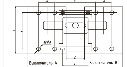
Установочные размеры механической блокировки
