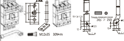
Минимальные размеры автоматических выключателей NM1-1250
