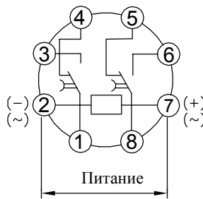
Рис. 9. Схема подключения JSZ3F-2Z
