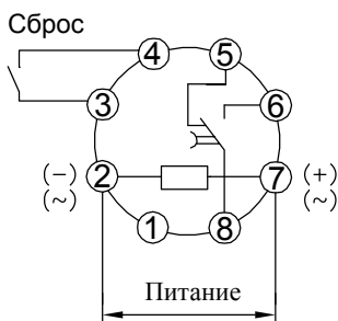
Рис. 8. Схема подключения JSZ3F
