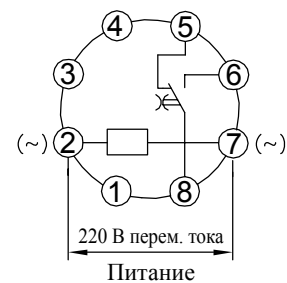
Рис. 22. Схема подключения JSZ3R (220 В)
