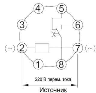
Рис. 22: Схема проводных соединений JSZ3R (220 В)
