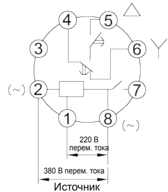
Рис. 16: Схема проводных соединений JSZ3Y (380 В, 220 В)
