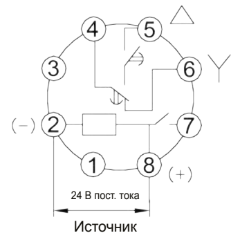
Рис. 19: Схема проводных соединений JSZ3Y (24 В пост. тока)
