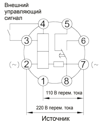
Рис. 10. Схема проводных соединений JSZ3K (220В, 110 В)
