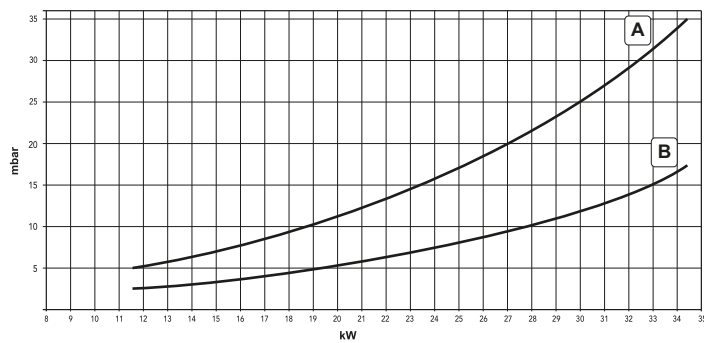
Diagrammi pressione - potenza DIVAtech D HF32
