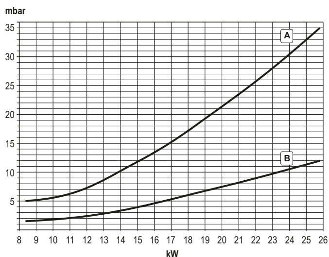
Diagrammi pressione - potenza DIVAtech D HF24
