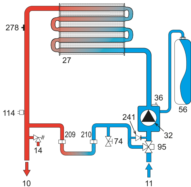
рис. 29- Контур отопления
