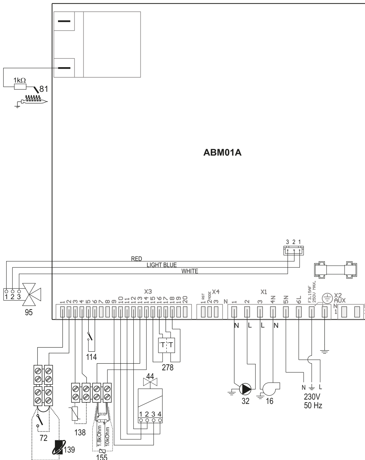
рис. 30- Электрическая схема
