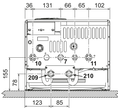
рис. 25- Вид снизу - HF24 и HF32
