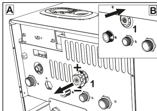
fig. 8- Filling knob
