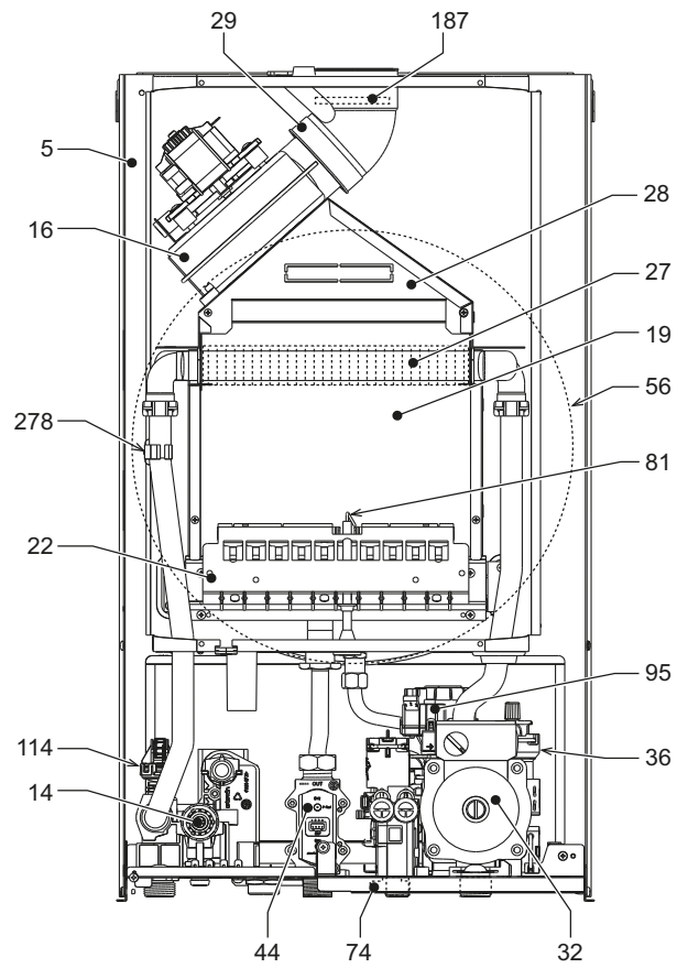
fig. 27- Vue générale - DIVAtech D HF24
