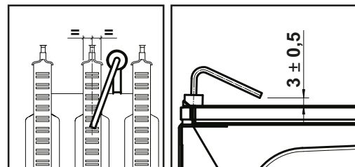
рис. 20 - Положение электрода
