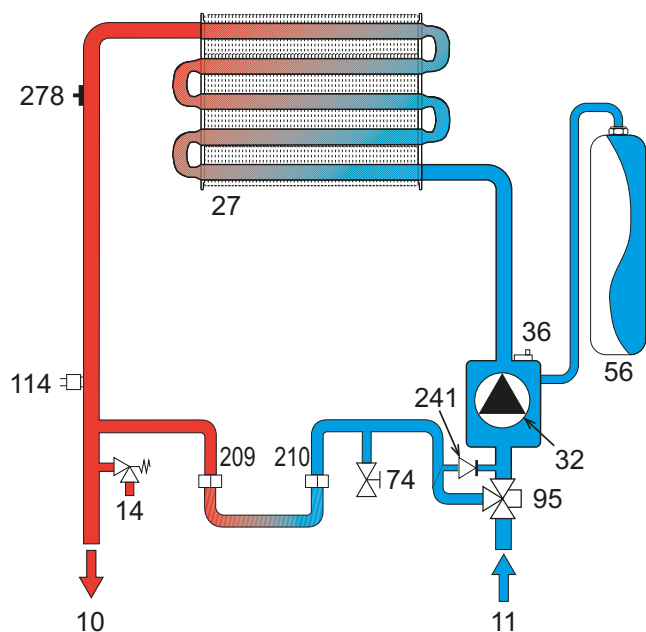
fig. 29- Circuit chauffage
