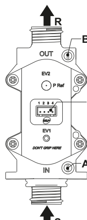
рис. 17 - Газовый клапан
