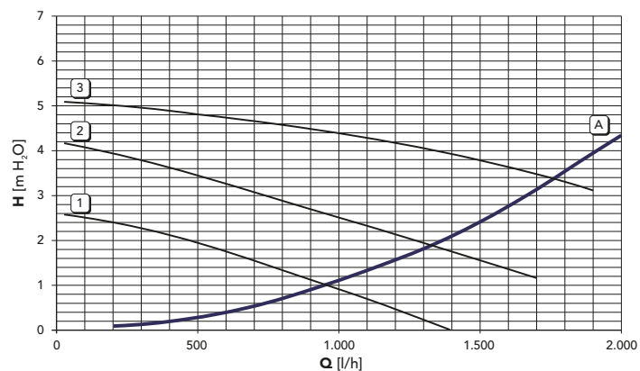
Perdite di carico / prevalenza circolatori DIVAtech D HF24
