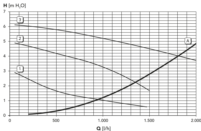
Perdite di carico / prevalenza circolatori DIVAtech D HF32
