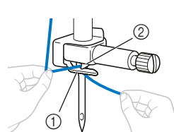
① Нитенаправитель игловодителя ② Язычок
