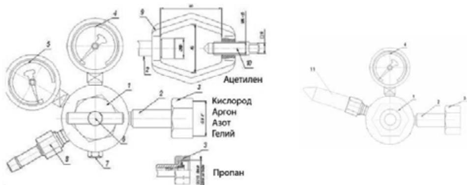
Рис. 1. Редуктор.
