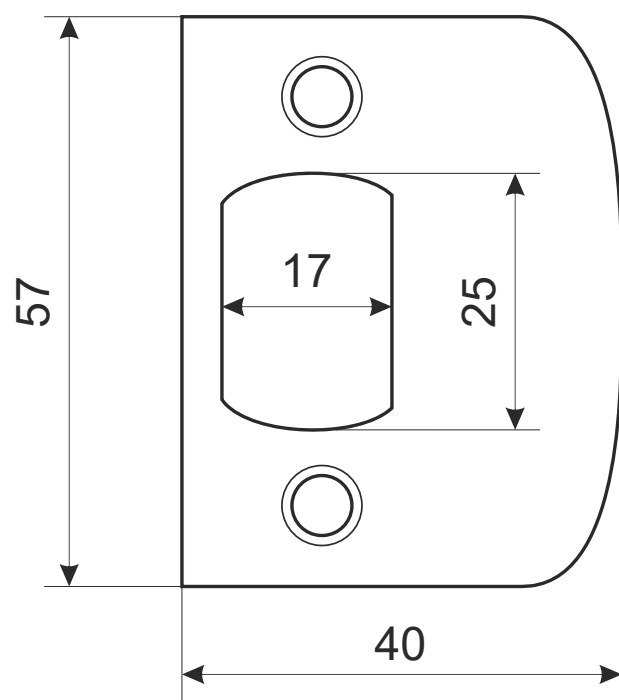
Ответная планка
