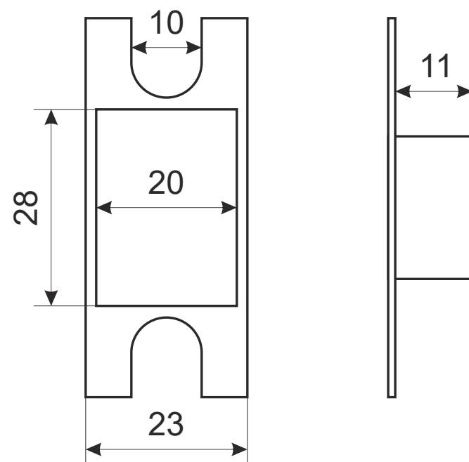
Пластиковая вставка
