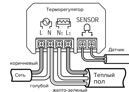
Подключение к 2-х проводной линии
