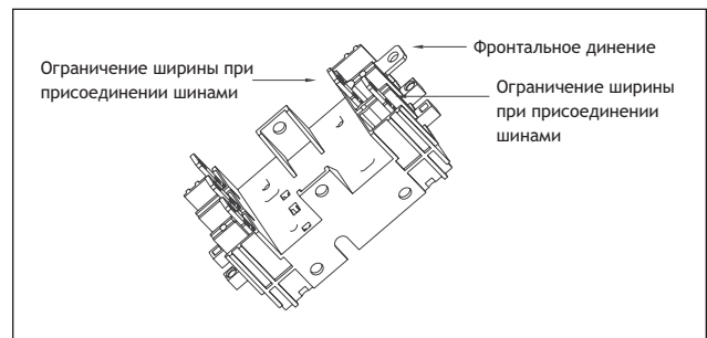
Втычное исполнение
