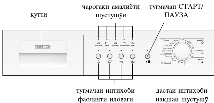
Расми 1 – Қисми идоракуни
