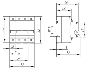
Рис. 1 Габаритные и установочные размеры ВН-29
