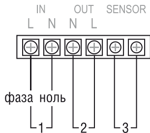
Пример подключения соединительных проводов к терморегулятору CALEO Model 320
