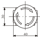
Рисунок 4. NP2-BS5□□
