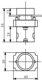
Рисунок 1. NP2-B A□□
