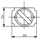
Рисунок 3. NP2-BD□□
