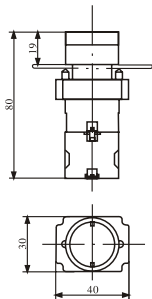
Рисунок 6. NP2-BW3□6, BW3□7
