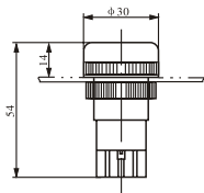
Рисунок 7. NP2-EV16□
