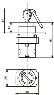
Рисунок 5. NP2-BG□□
