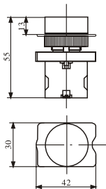
Рисунок 2. NP2-EA□□
