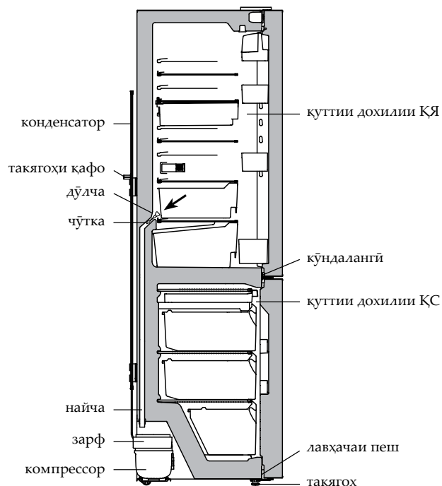
Расми 9 – Нақшаи резини яҳоба аз ҚЯ
