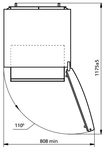
Şəkil 2 – Soyuducu (üstən görünüş)
