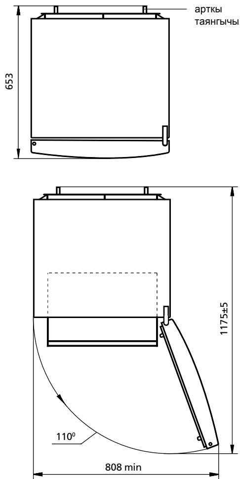
2-сүрөт – Муздаткыч (жогору жагынан көрүнгөн көрүнүшү)
