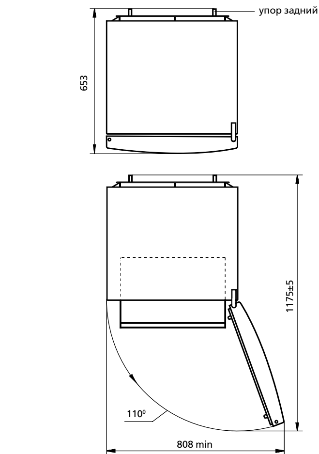
Рисунок 2 – Холодильник (вид сверху)
