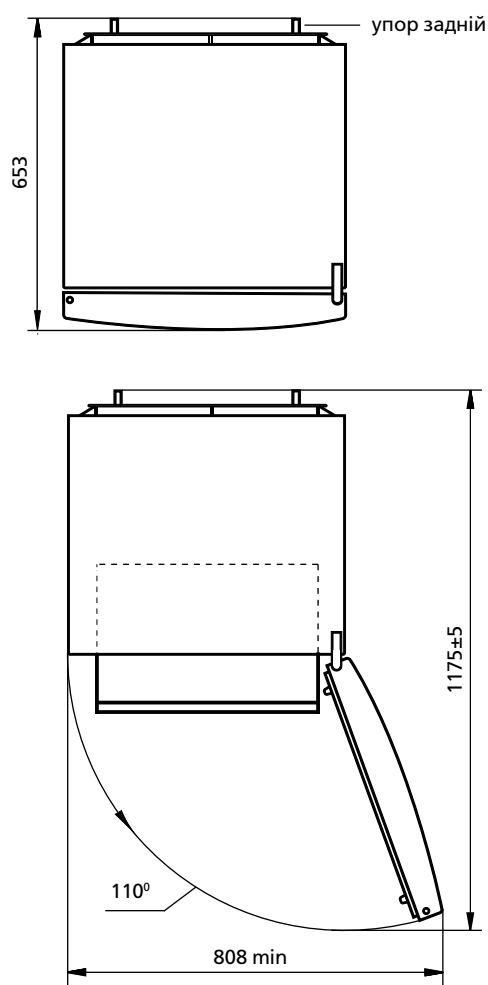
Малюнок 2 – Холодильник (вид зверху)
