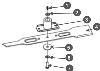
Рис. 27 Установка ножа
