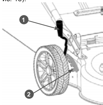
Рис. 18 Регулировка высоты кошения
