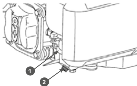
Рис. 25 Слив топлива из карбюратора 1. Карбюратор
