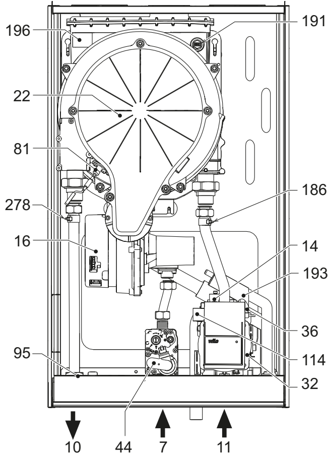
fig. 26 - Vista general
