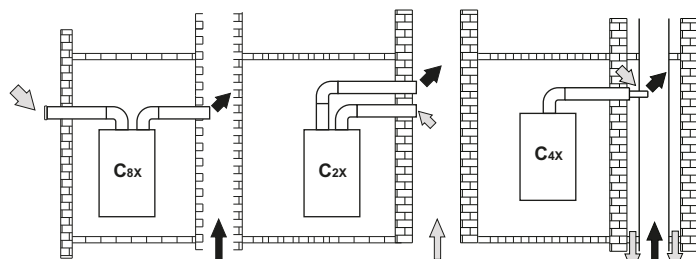
fig. 19 - Exemples de raccordement à des carneaux de fumées (⇨ = Air / ⇩ = Fumées)
