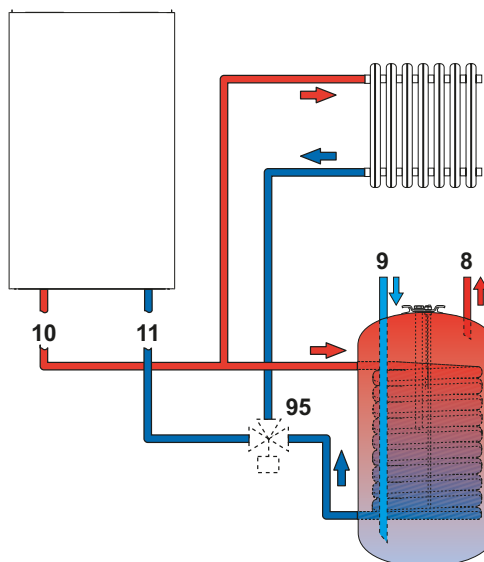
рис. 13 - Схема соединений с внешним бойлером
