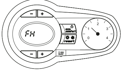
şek. 6 - Hava tahliye döngüsü
