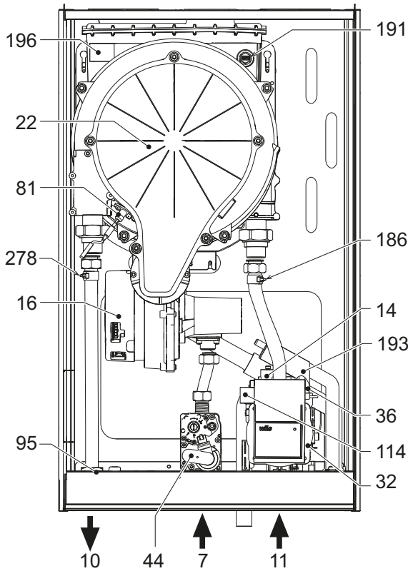
рис. 26 - Общий вид
