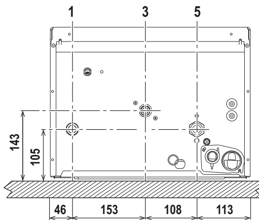
fig. 12 - Attacchi idraulici
