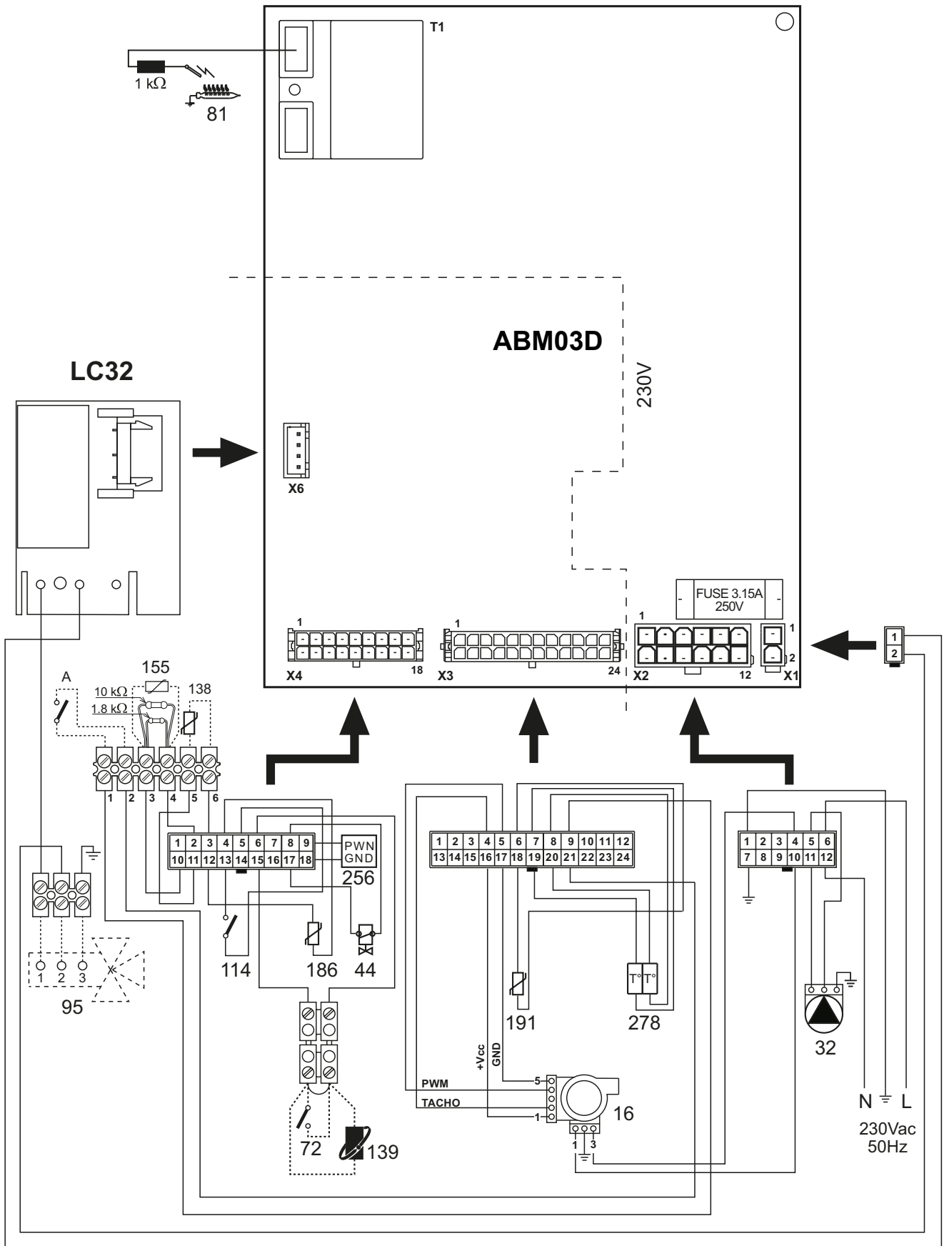
fig. 29 - Schéma électrique
