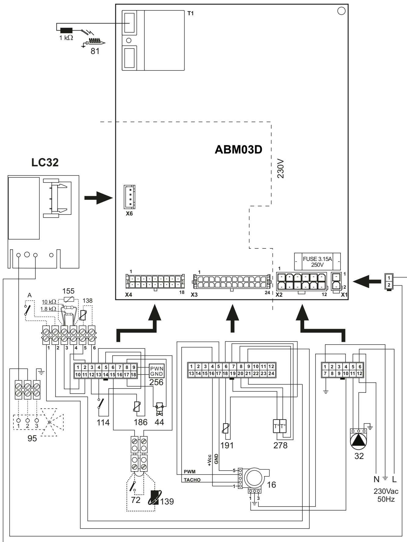
fig. 29 - Esquema eléctrico
