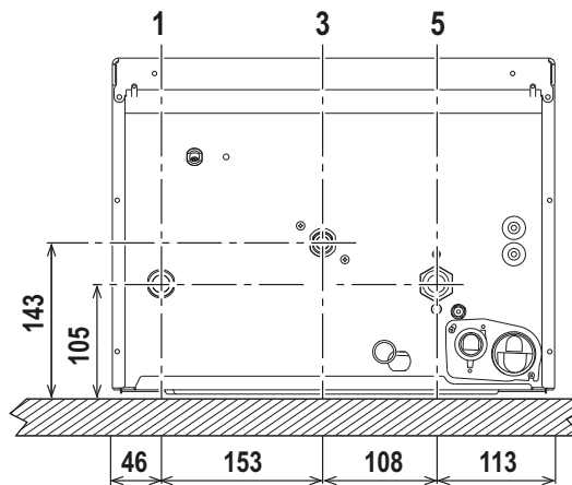
fig. 12 - Racorduri hidraulice
