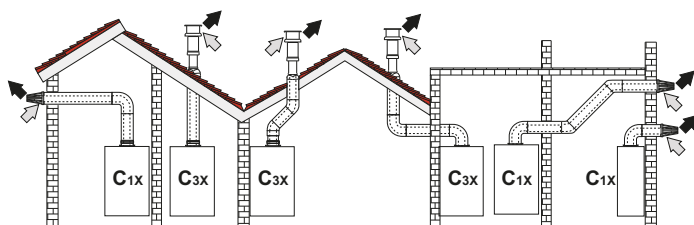
мал. 15 - Приклад підключення за допомогою співвісних (коаксимальних) труб (☞ = Повітря / ☛ = Відпрацьовані гази)
