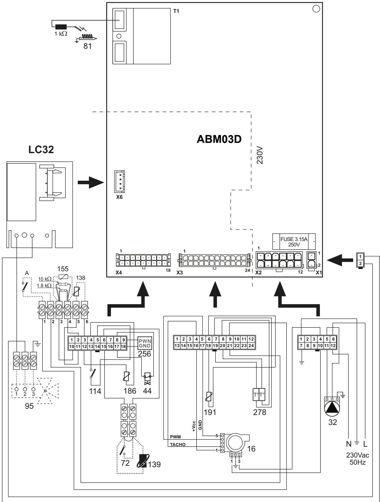
fig. 29 - Schema elettrico
