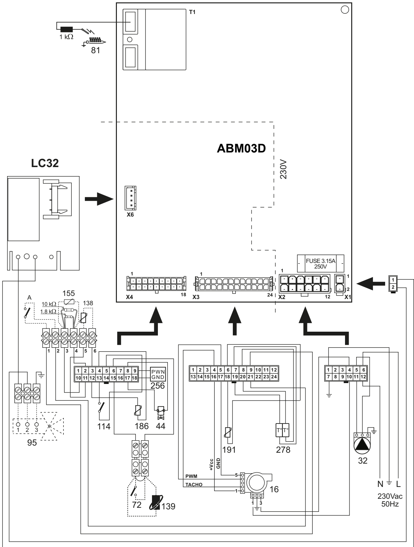
рис. 29 - Электрическая схема
