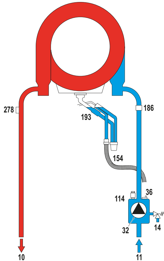
fig. 28 - Circuit hydraulique
