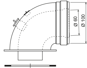
şek. 16 - Koaksiyal kanallar için çıkış aksesuarları
