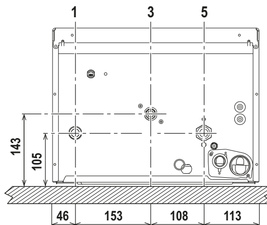
fig. 12 - Conexiones hidráulicas
