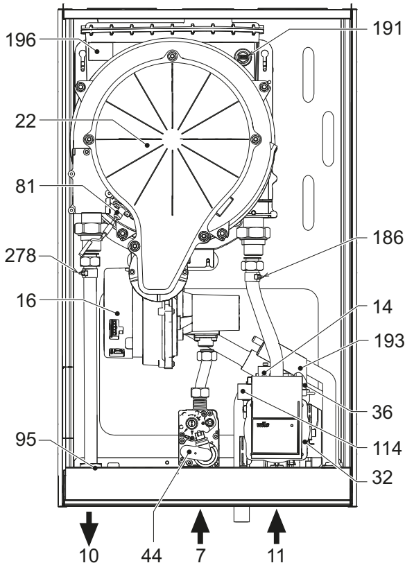
fig. 26 - Vue générale
