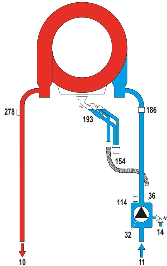
fig. 28 - Circuito hidráulico
