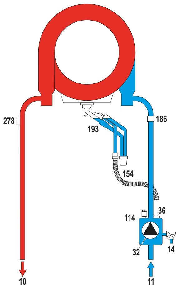
fig. 28 - Circuito idraulico
