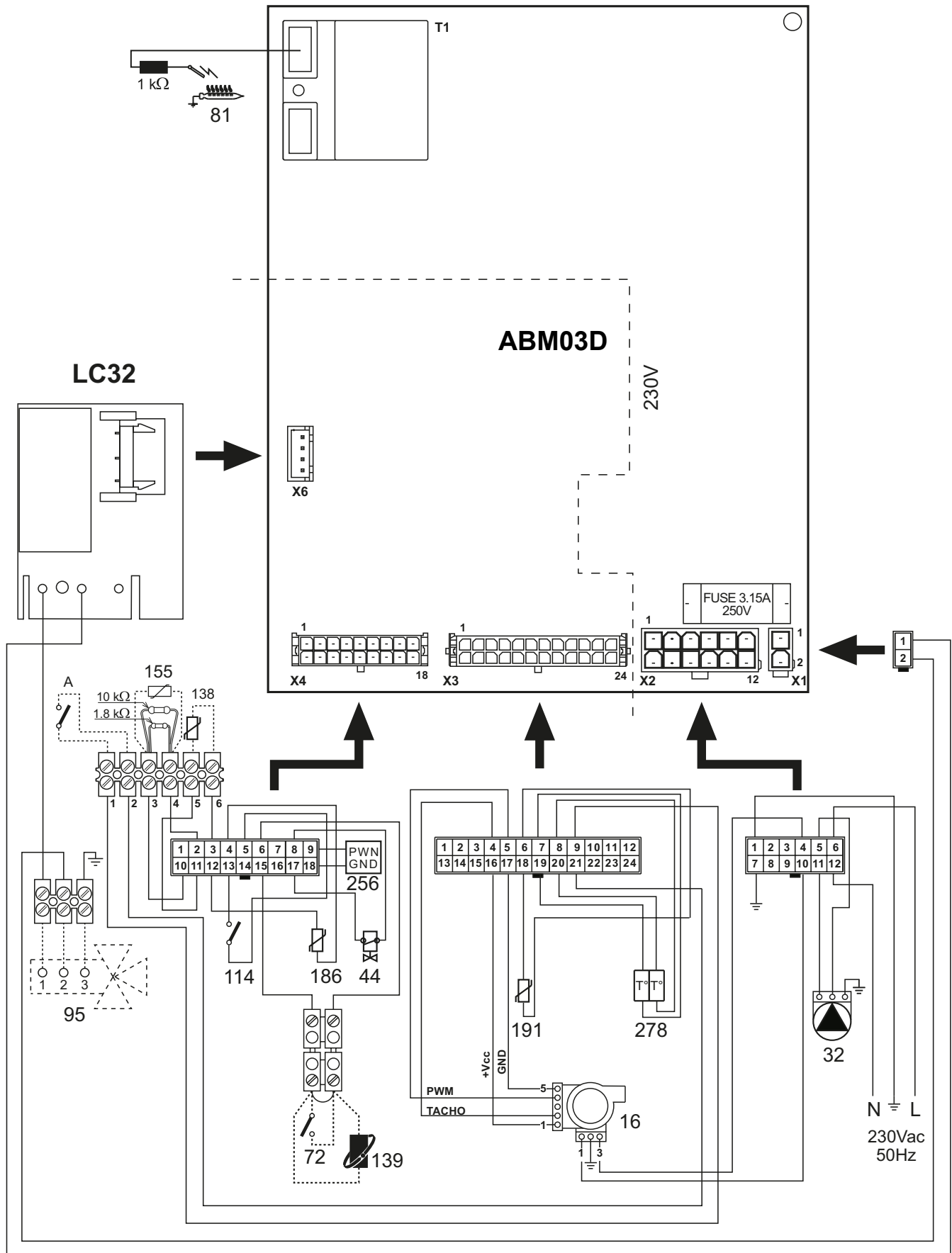
fig. 29 - Schemă electrică
