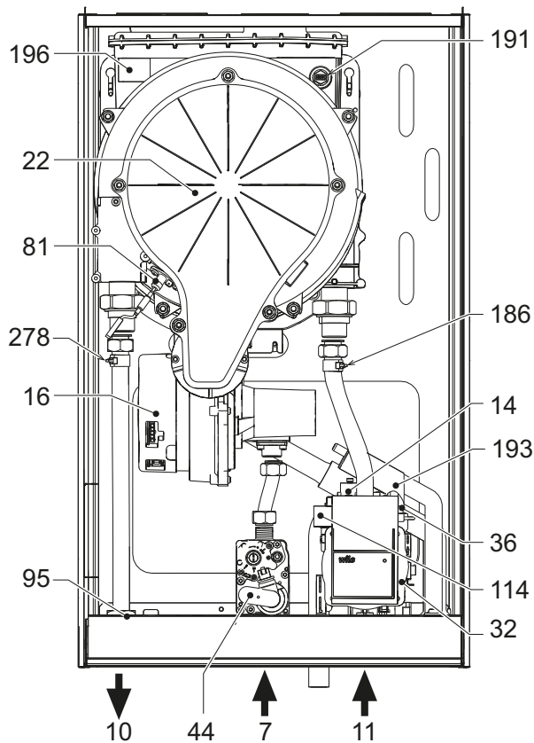
fig. 26 - Vedere generală
