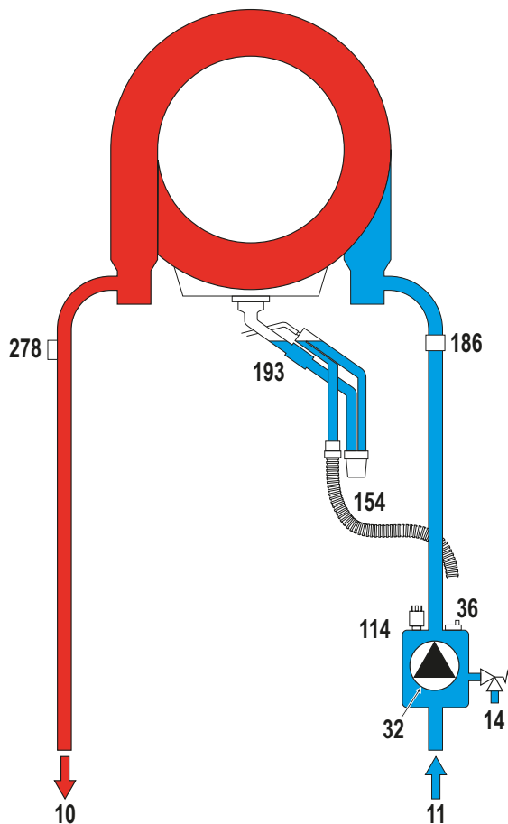
fig. 28 - Circuitul hidraulic
