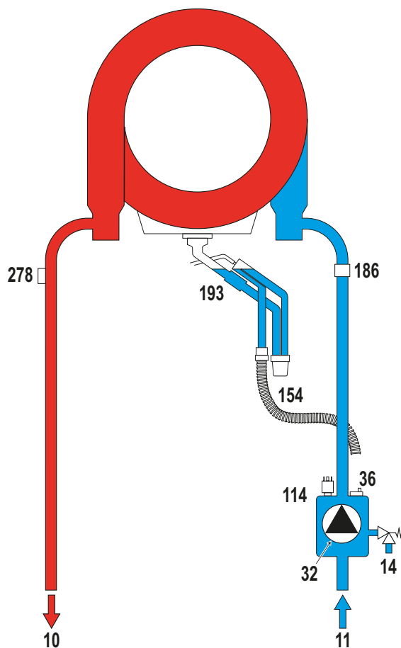
мал. 28 - Гідравлічний контур
