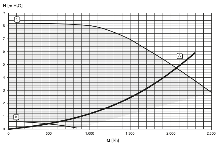
fig. 27 - Pertes de charge / pression circulateur
