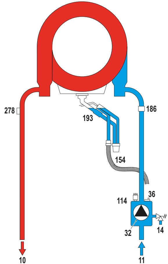
рис. 28 - Гидравлический контур
