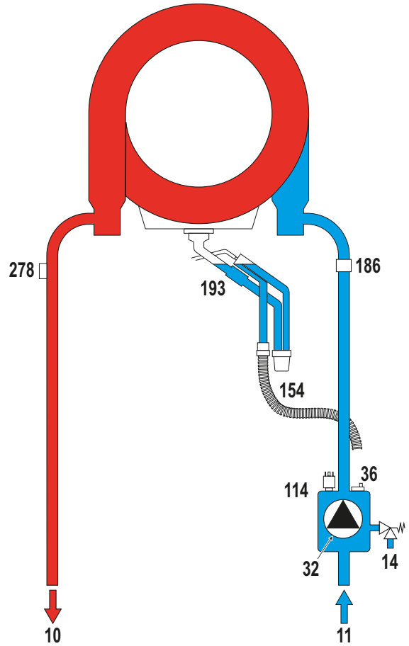
şek. 28 - Hidrolik devre
