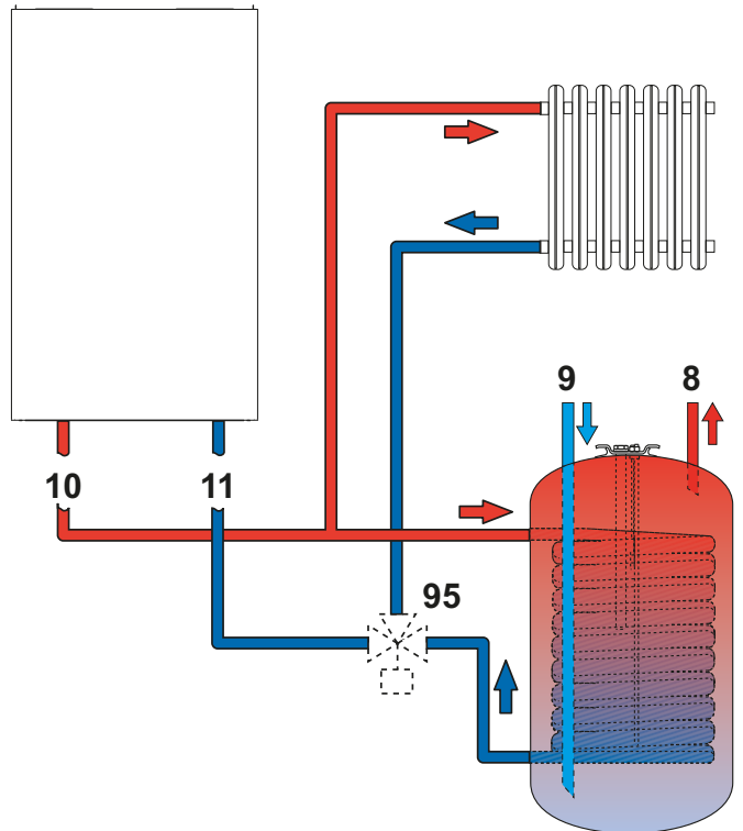
мал. 13 - Схема під'єднання до зовнішнього бойлера
