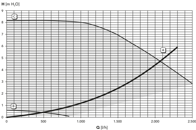
fig. 27 - Pérdidas de carga/altura manométrica circulador
