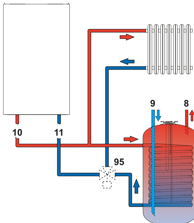
fig. 13 - Schéma de raccordement à un ballon extérieur
