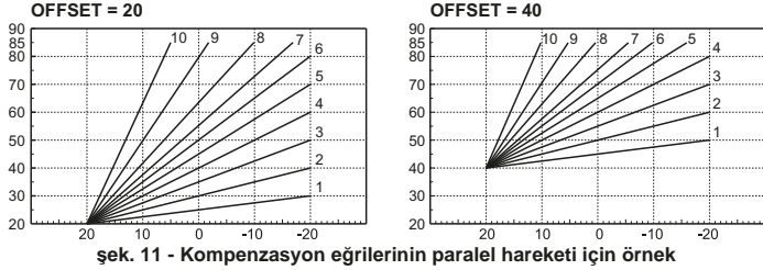
şek. 11 - Kompensasyon eğrilerinin paralel hareketi için örnek
