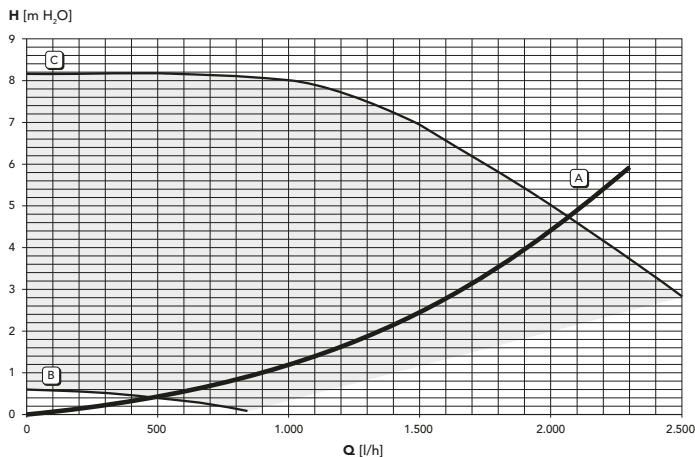
рис. 27 - Потеря напора/Напор циркуляционного насоса
