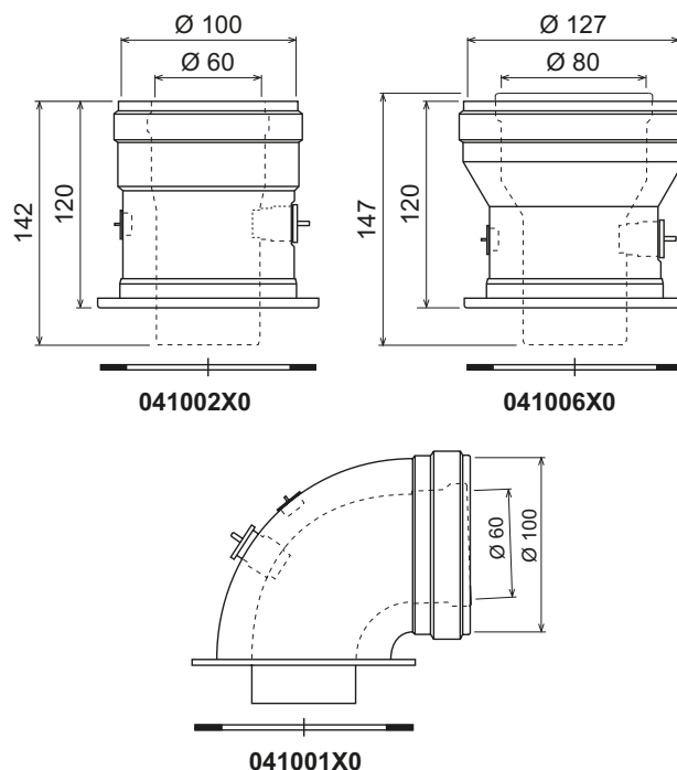
мал. 16 - Початкові елементи для коаксимальних трубопроводів
