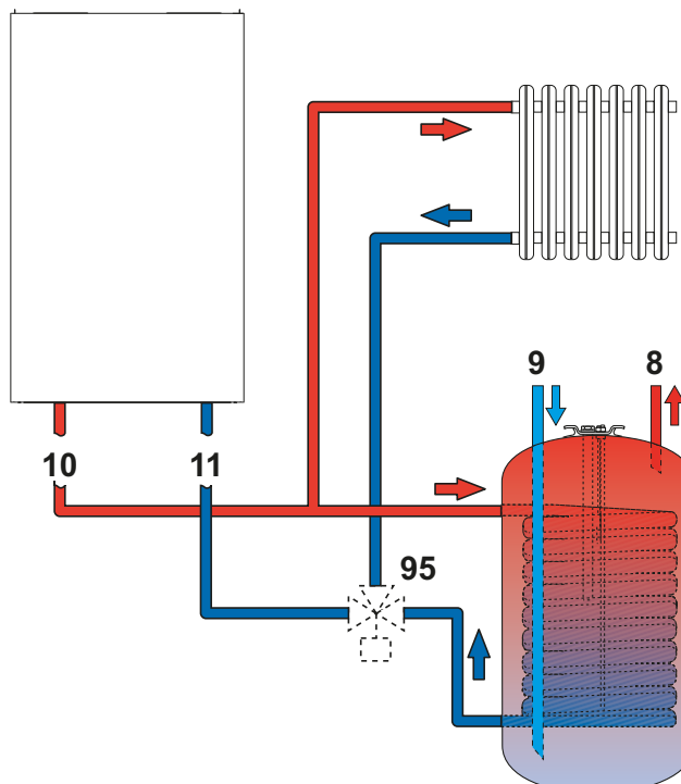
fig. 13 - Esquema de conexión a un acumulador externo
