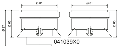
рис. 18 - Соединительный элемент для раздельных труб
