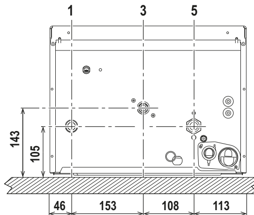
рис. 12 - Гидравлические соединения
