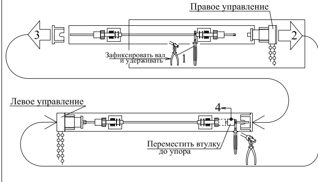
ВИД СВЕРХУ НА КАРНИЗ
