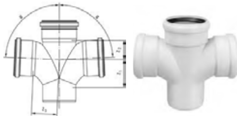
SKDA – крестовина 87°
