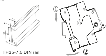
TH35-7.5 DIN rail
