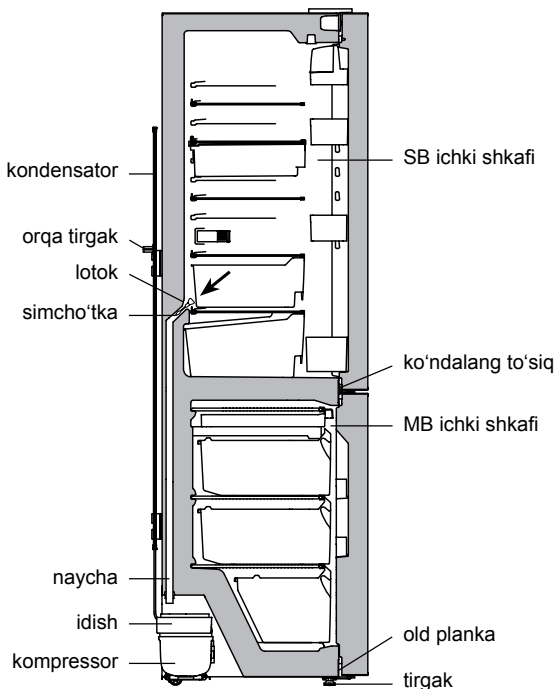
9-rasm – SB erigan suvni oqizish chizmasi
