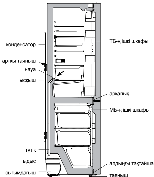
9-сурет – ТБ-тен жайылма су ағу сызбасы
