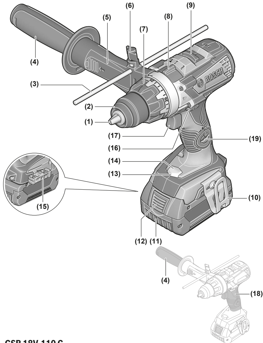
GSB 18V-110 C
