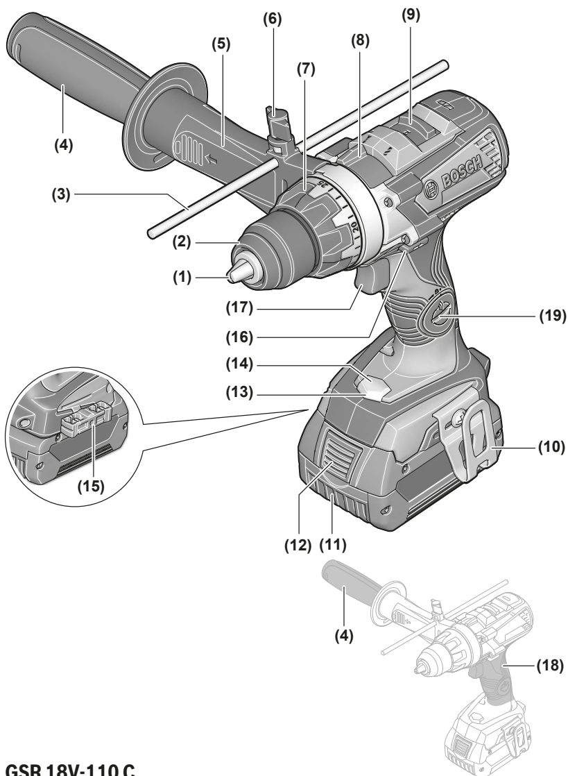
GSR 18V-110 C
