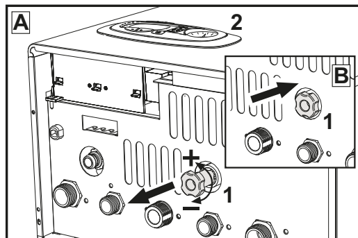
fig. 8- Robinet de remplissage
