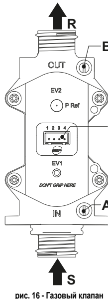
рис. 16 - Газовый клапан
