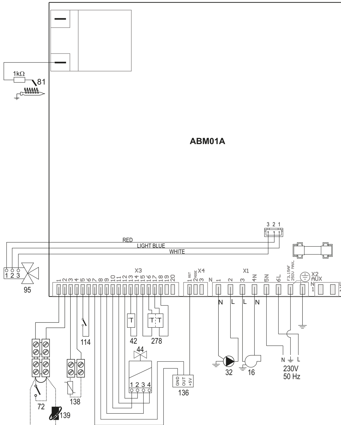
рис. 31- Электрическая схема
