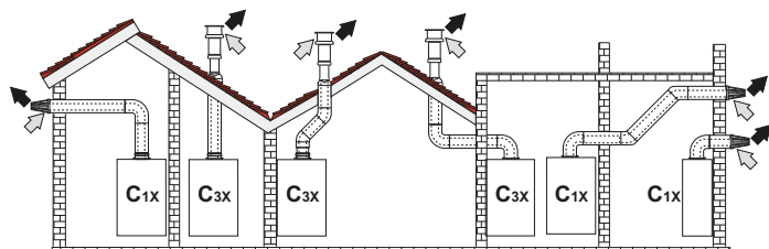
fig. 11 - Exemples de raccordement avec des conduits coaxiaux (⇨ = Air / ⇨ = Fumées)
