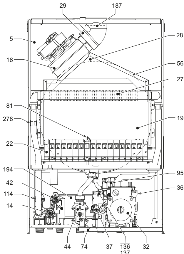
fig. 29- Vue générale - DIVAtech D F37
