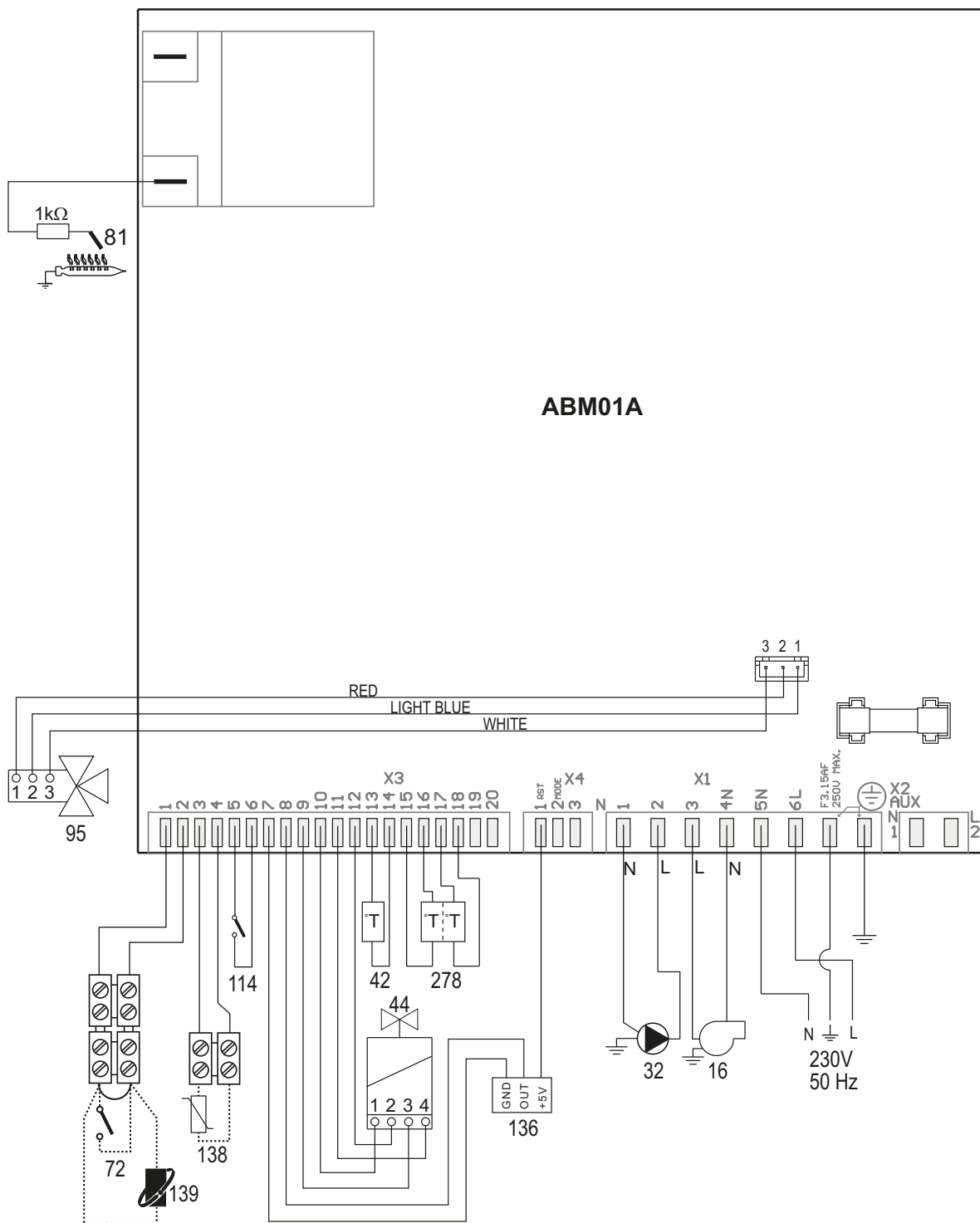
fig. 31- Wiring diagram
