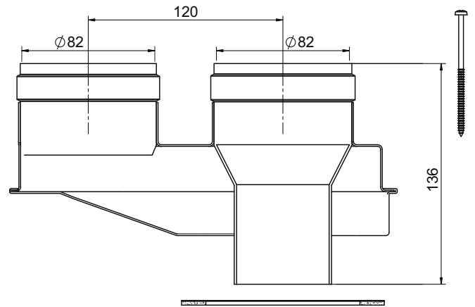
рис. 14- Исходная деталь для отдельных труб, код 010031X0
