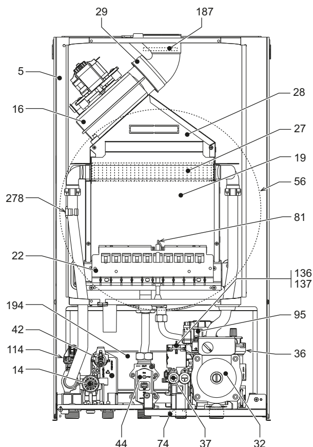
fig. 27- Vue générale - DIVAtech D F24
