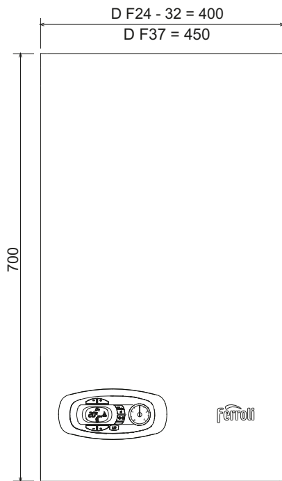
fig. 20- Vue de face
