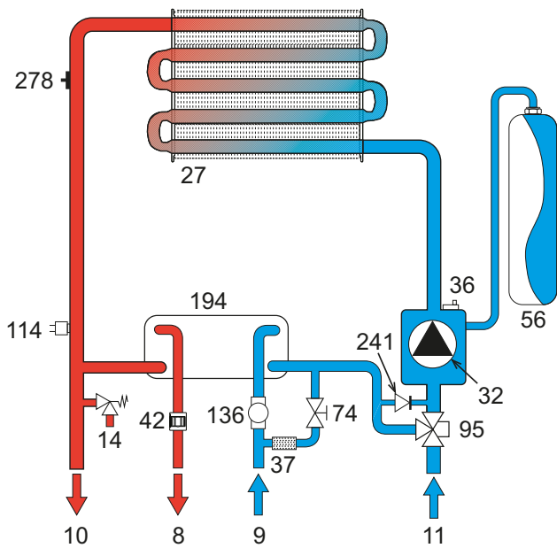
рис. 30- Контур отопления
