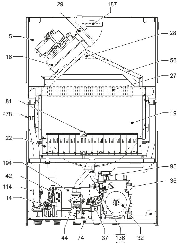
рис. 29- Общий вид - DIVAtech D F37
