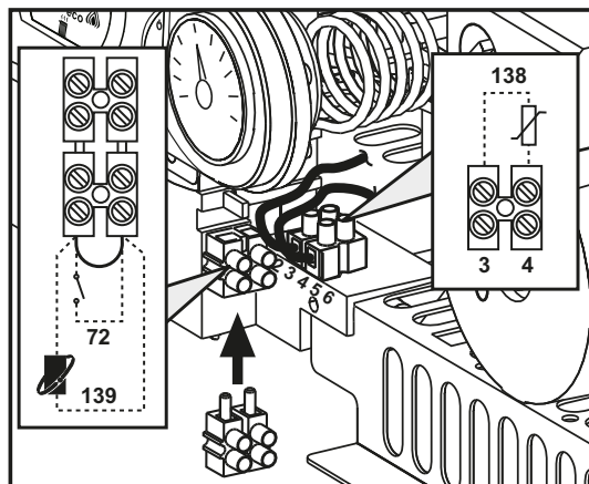
рис. 10 - Доступ к клеммной коробке
