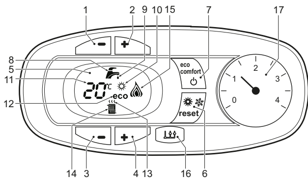
рис. 1 - Панель управления
