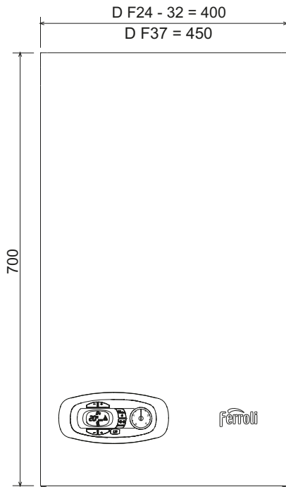
рис. 20- Вид спереди
