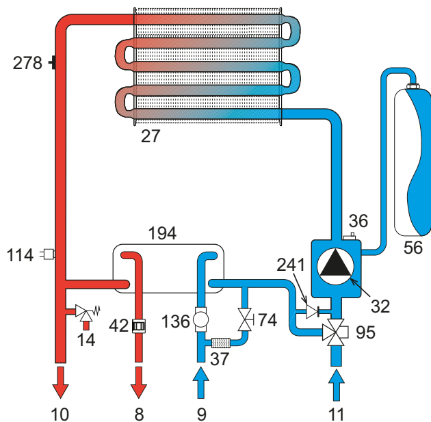
fig. 30- Circuit chauffage
