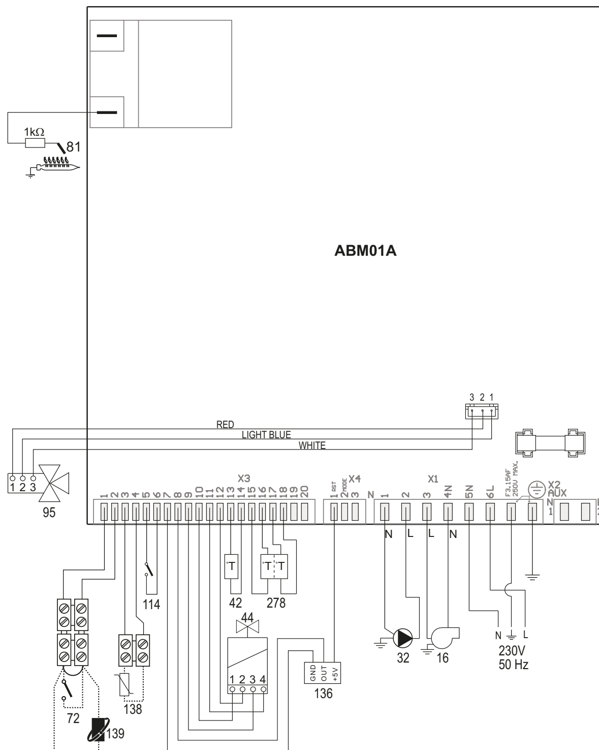
fig. 31- Schéma électrique
