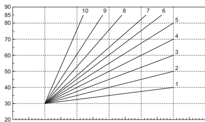
рис. 6 - Компенсационные характеристики
