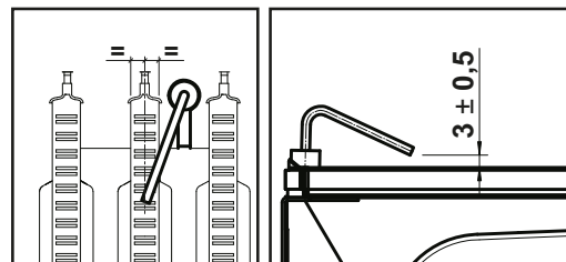
рис. 19 - Положение электрода
