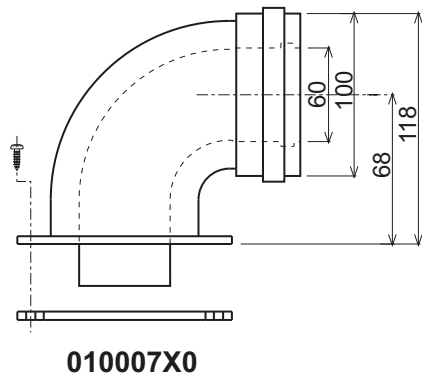
fig. 12 - Accessoires de départ pour conduits coaxiaux
