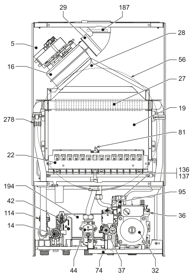
fig. 28- Vue générale - DIVAtech D F32
