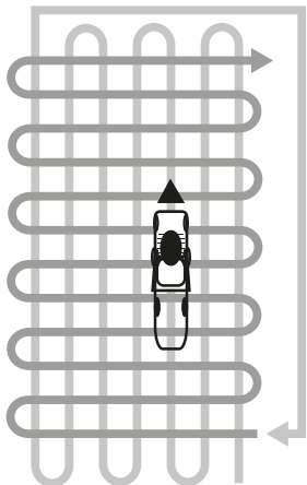
Рис. 14 Схема скашивания высокой и/или загущенной травы
