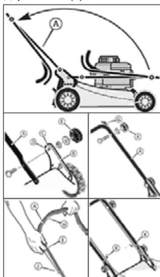
Рис. 2 Сборка газонокосилки
