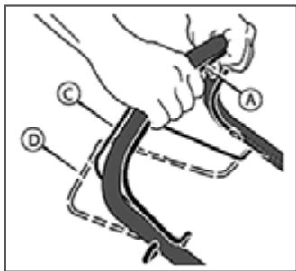
Рис. 13 Положение рычагов остановки двигателя и привода хода
