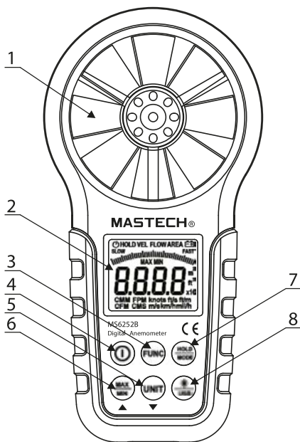
ПЕРЕДНЯЯ ПАНЕЛЬ
