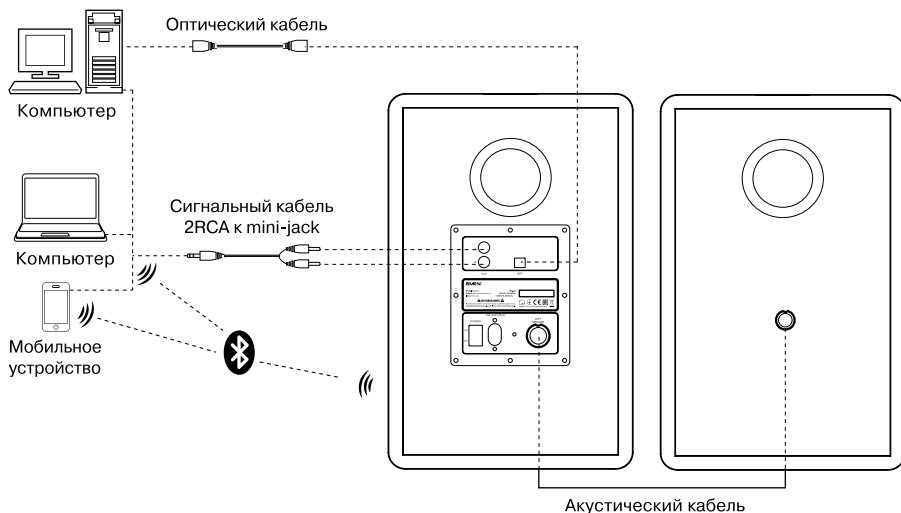
Рис. 4. Схема подключения
