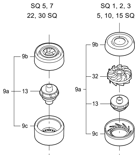
Рис. 4 Сборка камеры
