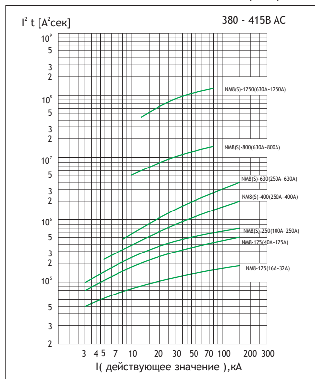
A^2сек характеристика
