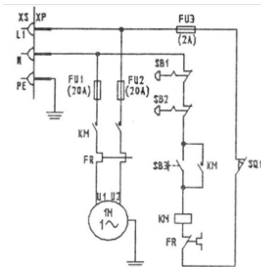
Электрическая схема
