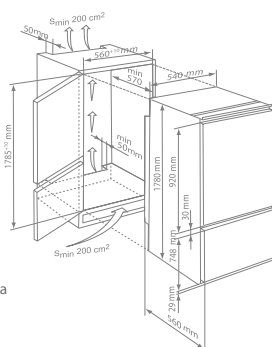
Схема встраивания холодильника ХМ-4307
