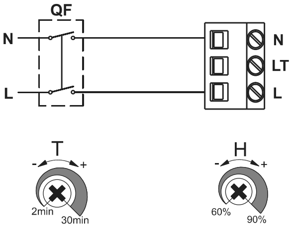
QF - автоматический выключатель
