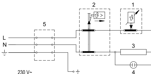
Šema povezivanja električnih provodnika
