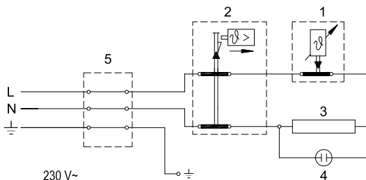
Электр тізбесінің схемасы
