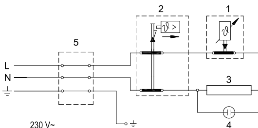
Електросхема
