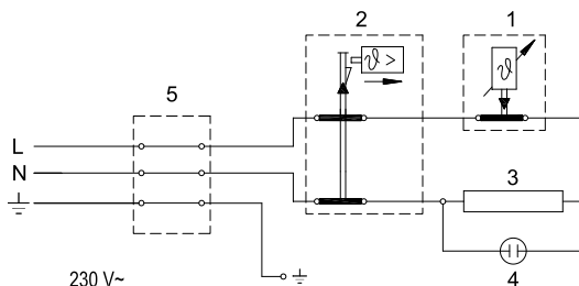
Instalația electrică
