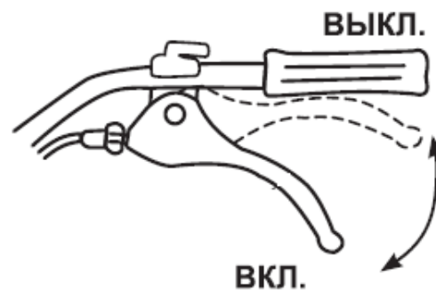
Рисунок 7 – Рычаг сцепления
