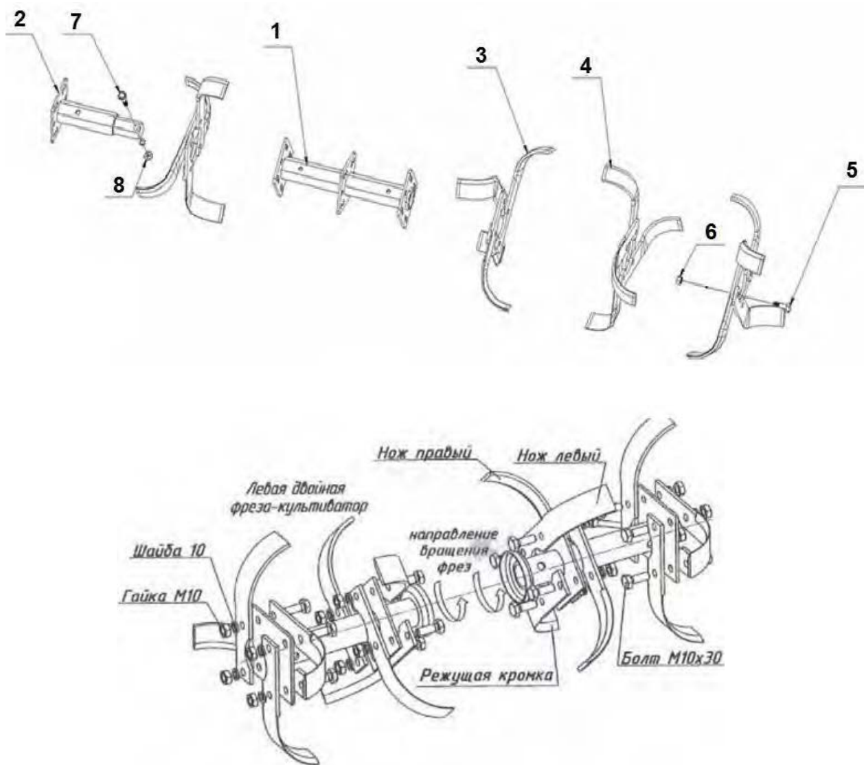
Рисунок 3 – Сборка фрез
