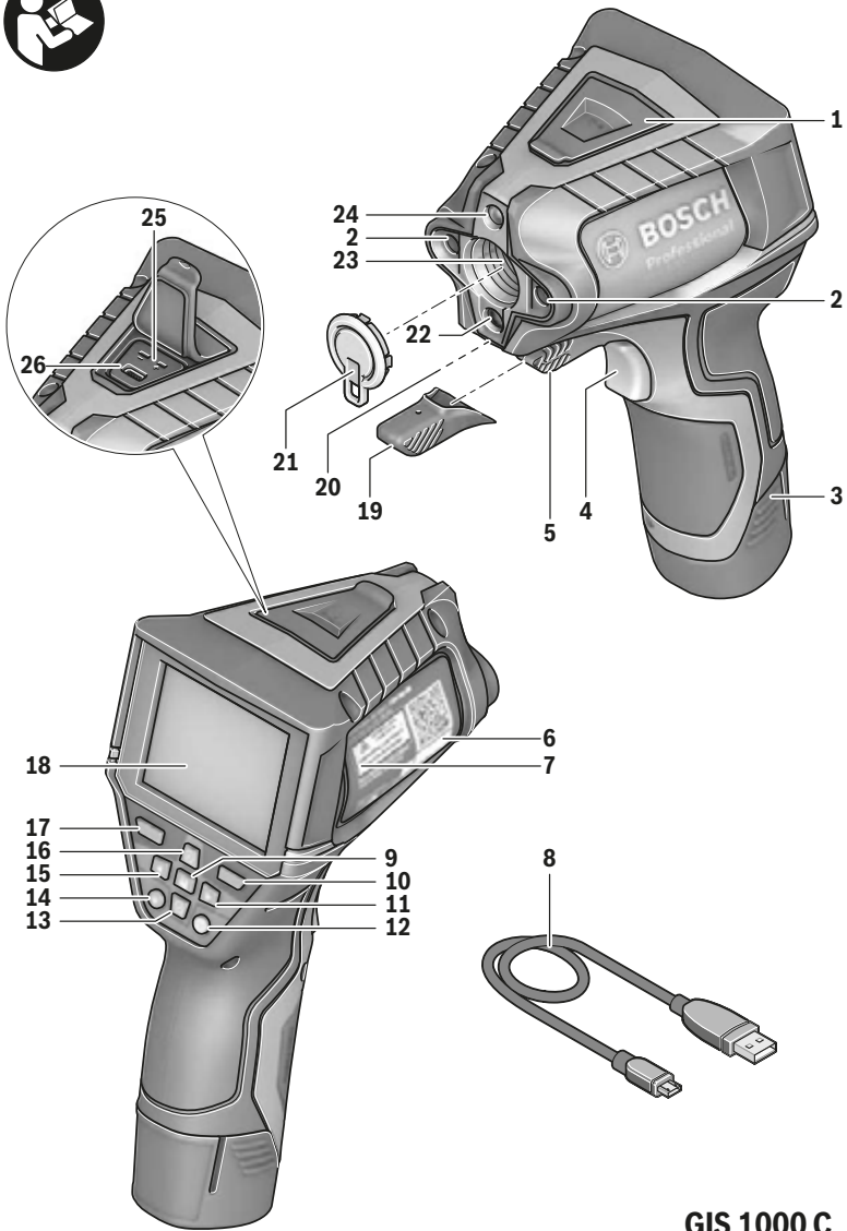
GIS 1000 C
